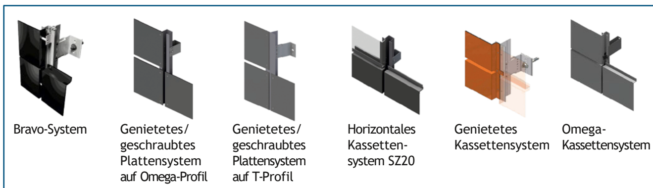
Abb. 14 - Fassadensysteme
