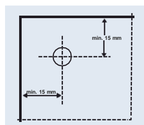
Abb. 6 - Randabstände
