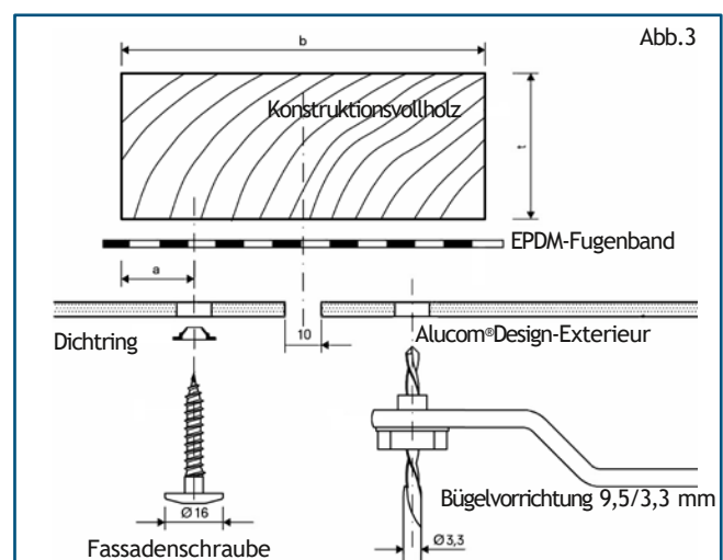
Abbildung - Mindestabmessungen der Traglattung nach DIN 1052
